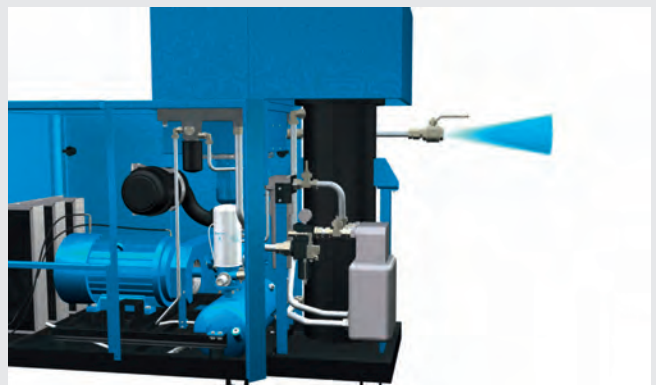
4. El aire BOGE producido está exento de aceite según la clase superior 0.
